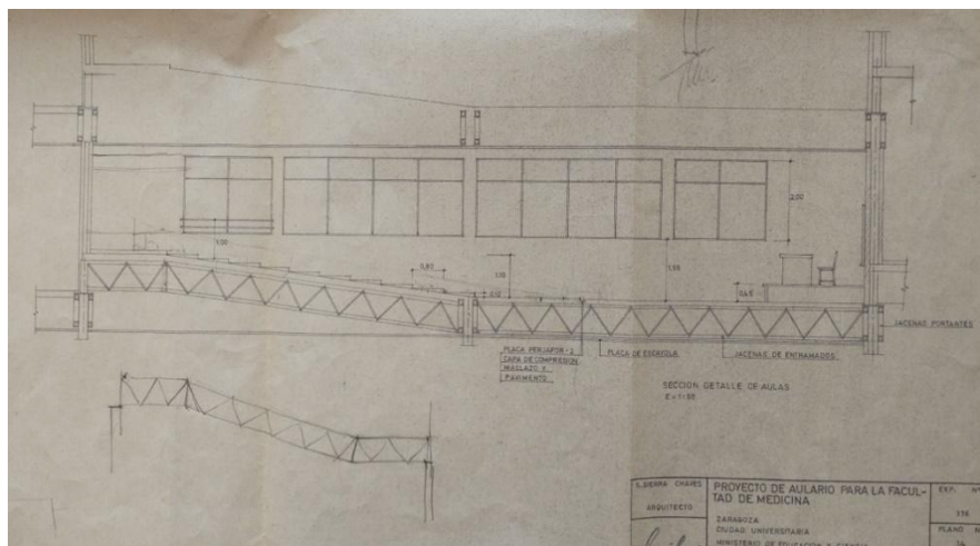
Imagen 4. Sección detalle de aulas. Fuente: Archivo UTCE.
