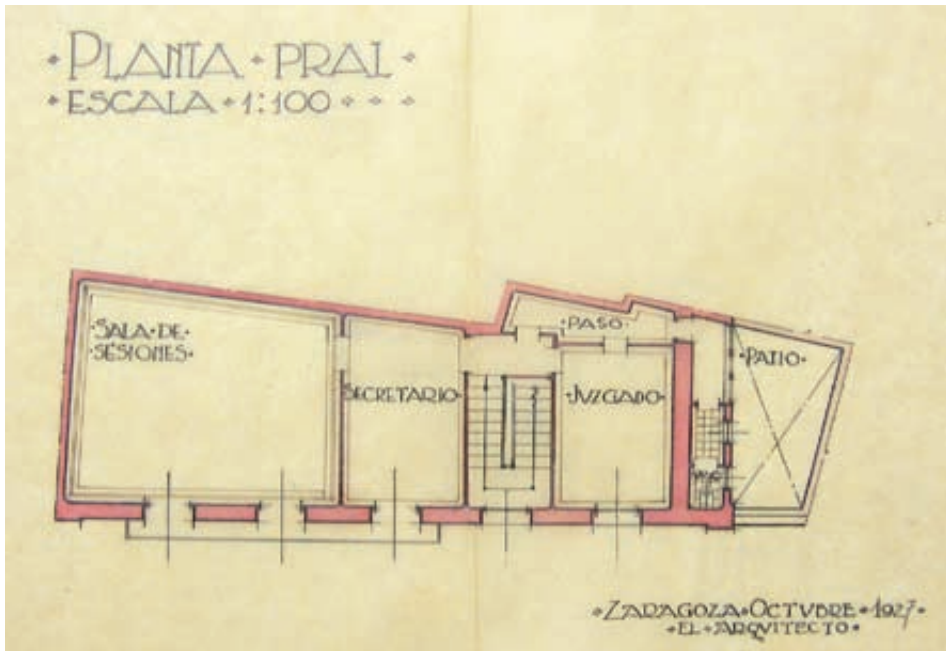
Fig. 11. Planta principal del anteproyecto de casa consistorial de Aguilón, 1927 (A.D.P.Z.).
