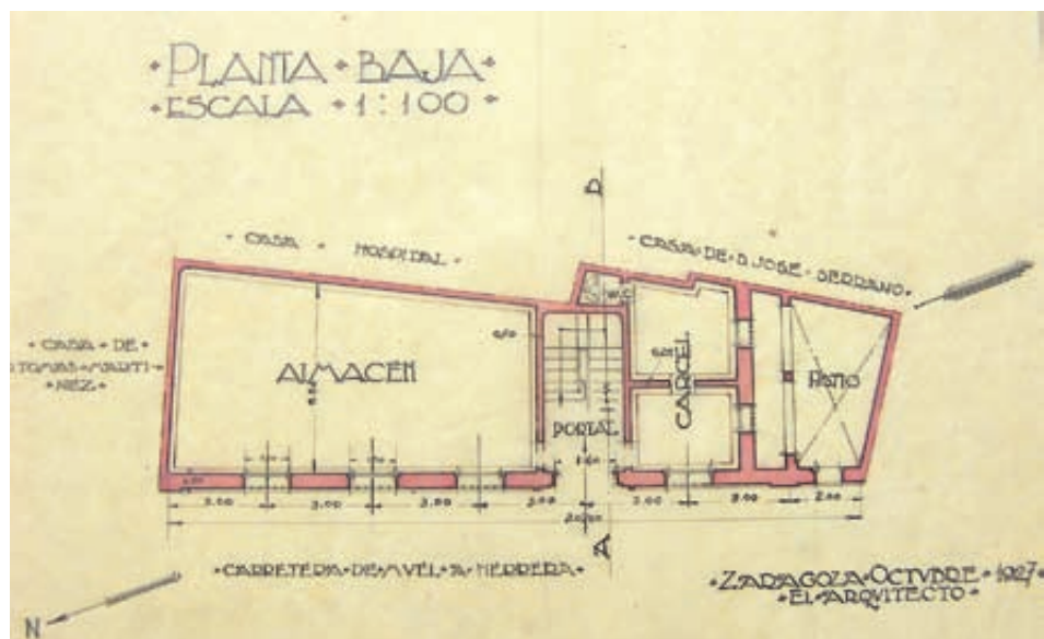
Fig. 10. Planta baja del anteproyecto de ayuntamiento de Aguilón, 1927 (A.D.P.Z.).
