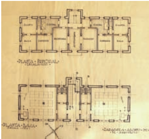
Fig. 6. Plantas baja y principal del proyecto de casa consistorial de Embid de la Ribera, 1924 (A.D.P.Z.).
