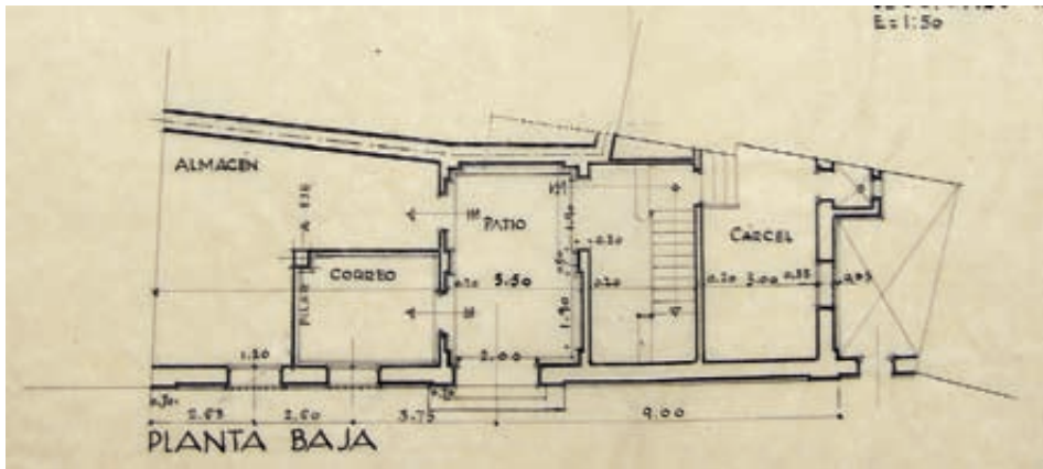
Fig. 13. Planta baja del proyecto de casa consistorial de Aguilón, 1929 (A.D.P.Z.).
