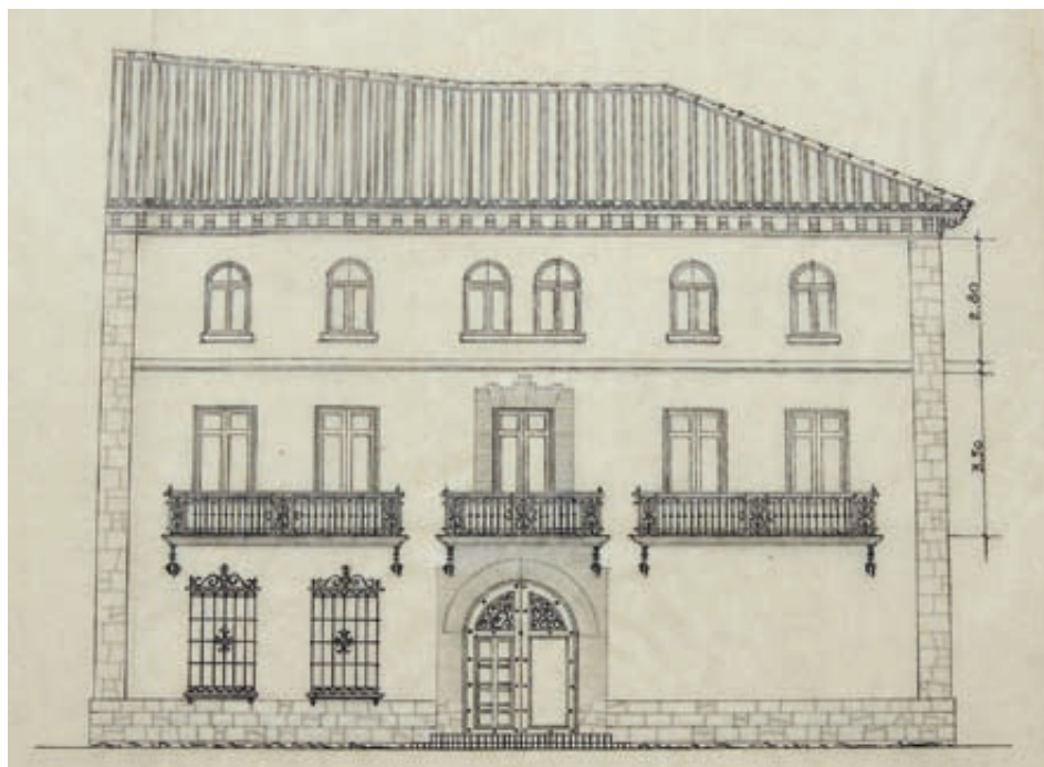
Fig. 14. Fachada principal del proyecto de ayuntamiento de Aguilón, 1930 (A.D.P.Z.).
