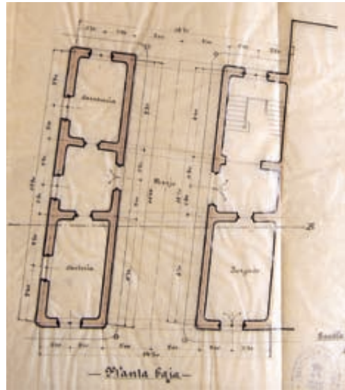
Fig. 2. Planta baja del proyecto de casa consistorial de Cosuenda, 1921 (A.D.P.Z.).
