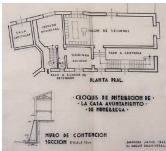
Fig. 18. Planta y sección del proyecto de consolidación del ayuntamiento de Munébrega, 1942 (A.D.P.Z.).
