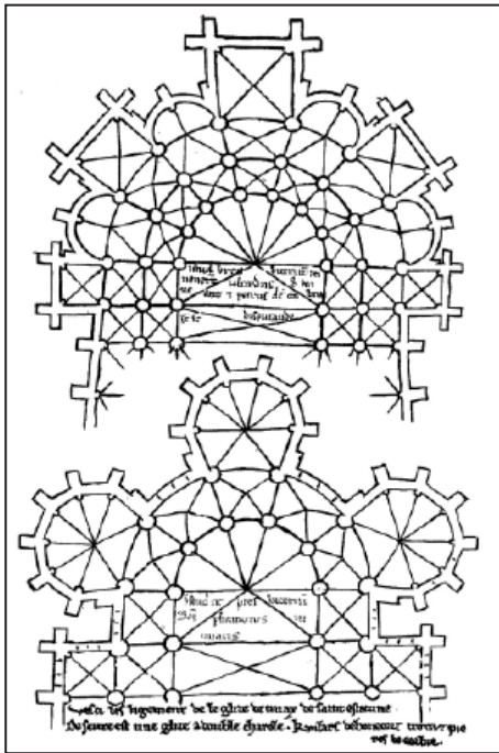
Fig. 1. Plantas de iglesias recogidas por Villard d'Honnecourt.
