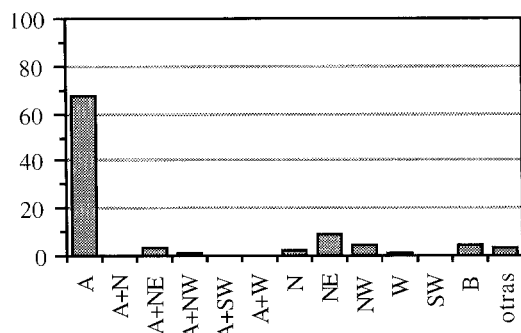
Figura 2.- Tipos de tiempo asociados a heladas. Valores porcentuales.
