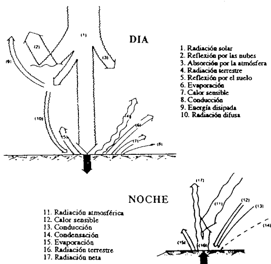
Figura 1.- Balance térmico tierra-atmósfera durante el día y la noche (URBANO, 1989).
