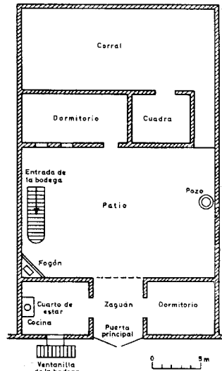
CASA RURAL MANCHEGA (Tomelloso, Ciudad Real)
