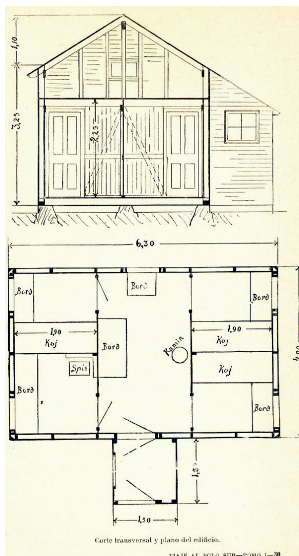
Figura 1. Corte transversal y plano de la cabaña de Nordenskjöld 1902-1904. Cfr. Otto Nordenskjöld. Viaje al Polo Sur. Expedición sueca a bordo del Antártico . (P.233). Barcelona 1904.
