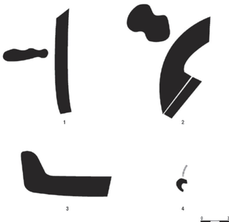
Figura 5. Cultura material recuperada en la excavación (1. asa de jarra; 2. asa de dolia; 3. tegulae y 4. lucerna).
