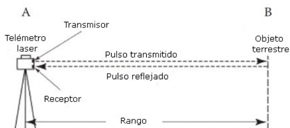
Figura 6. Funcionamiento básico de un Telémetro láser que utiliza el pulso TOF:
