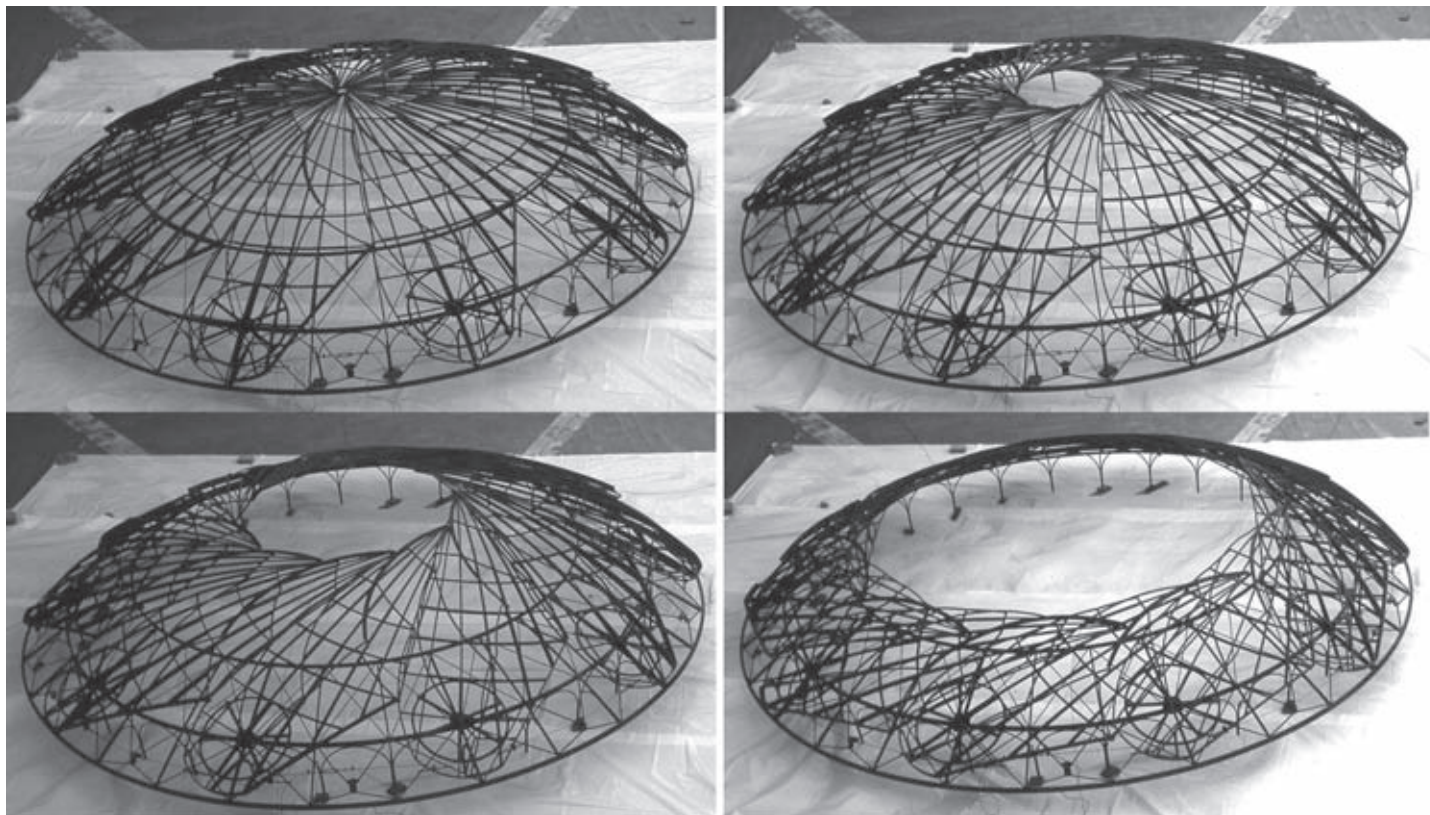
[Fig.5]. Emilio Pérez Piñero, Cúpula reticular practicable de directriz esférica, 1970. Fuente: Fundación Emilio Pérez Piñero.
